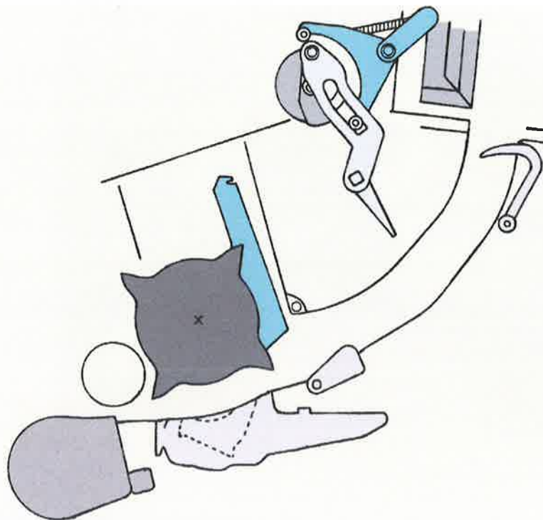
Afb. 4.8 Het gewas wordt door een rotor de voorperskamer ingevoerd.
