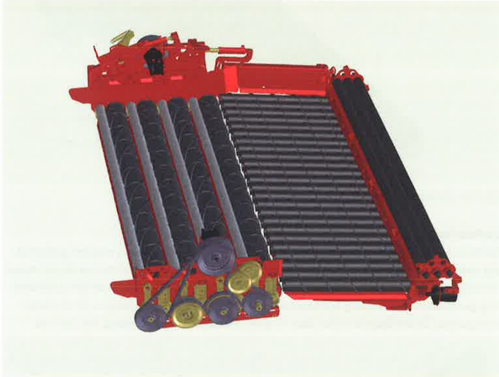
Afb. 5.18 De axiaalrollen verwijderen de nog overgebleven grond.
