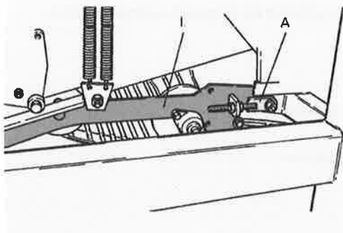
Afb. 5.33 Door de keerrrolsteun L te verschuiven met spanbout A span of ontspan je de zeefketting.
